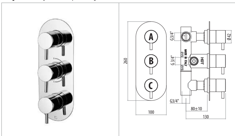
A. Apertura/Chiusura unica via di uscita Opening/Closing single outlet
