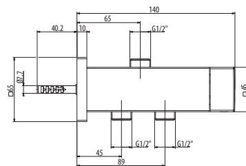
Desviador de pared de 2 vías
