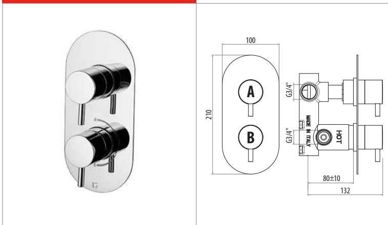
A. Apertura/Chiusura e deviazione 2 uscite separate Opening/Closing and diverting 2 split outlets
