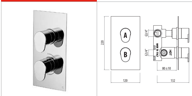
A. Apertura/Chiusura e deviazione 2 uscite separate Opening/Closing and diverting 2 split outlets
